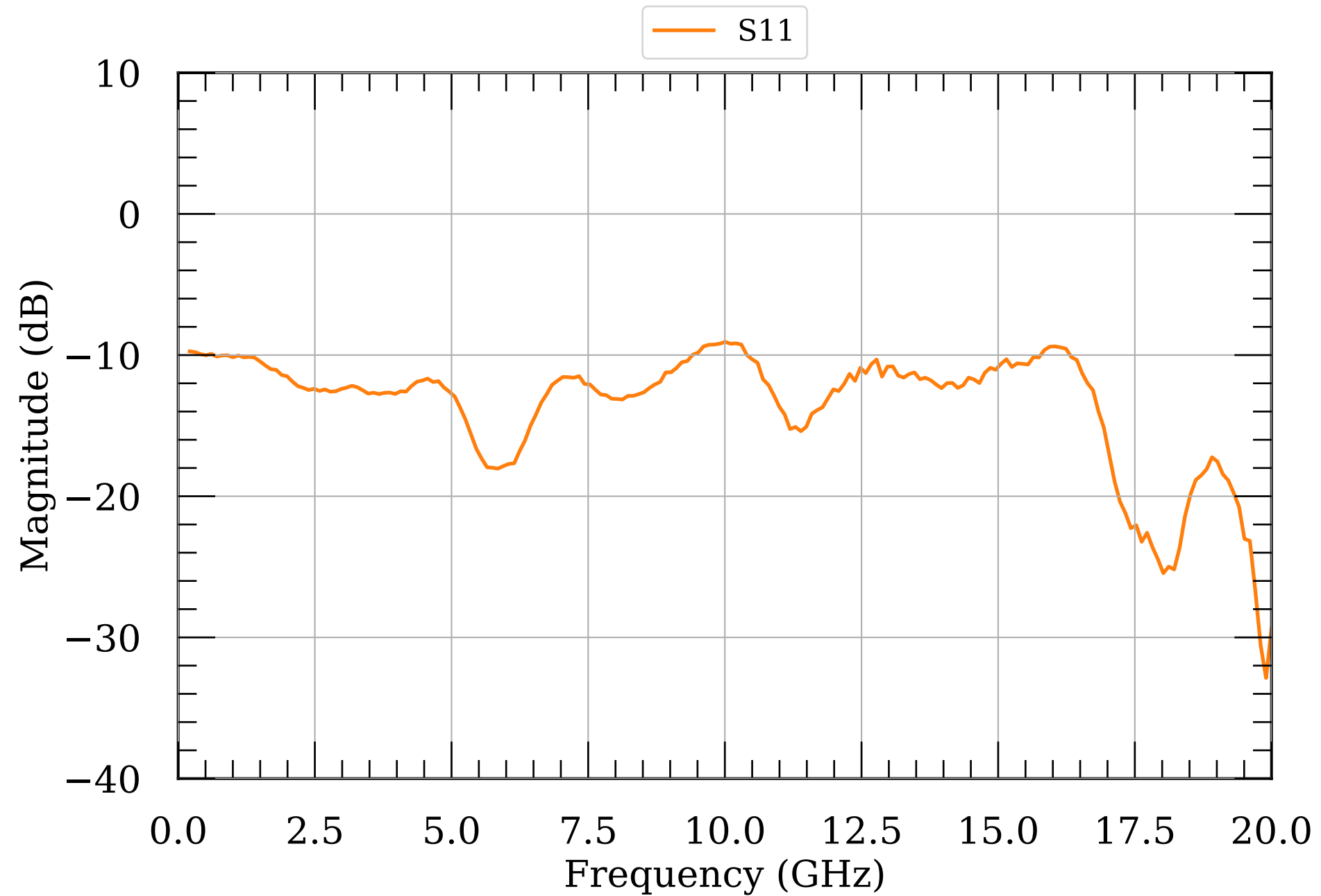
LNA S-params module002v3
